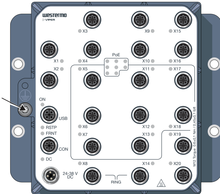
Abbildung 6. Erdungsanschluss
