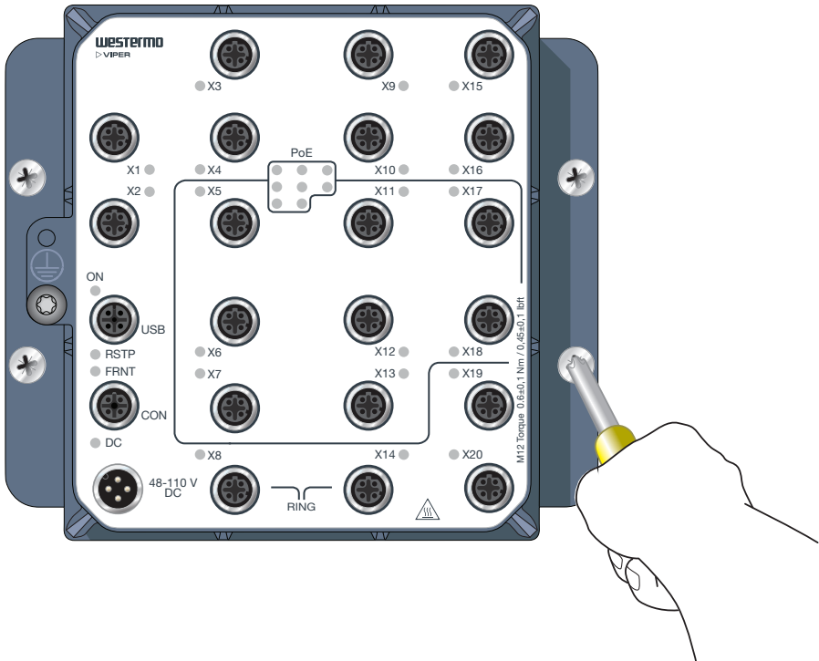
Abbildung 5. Wandmontage
