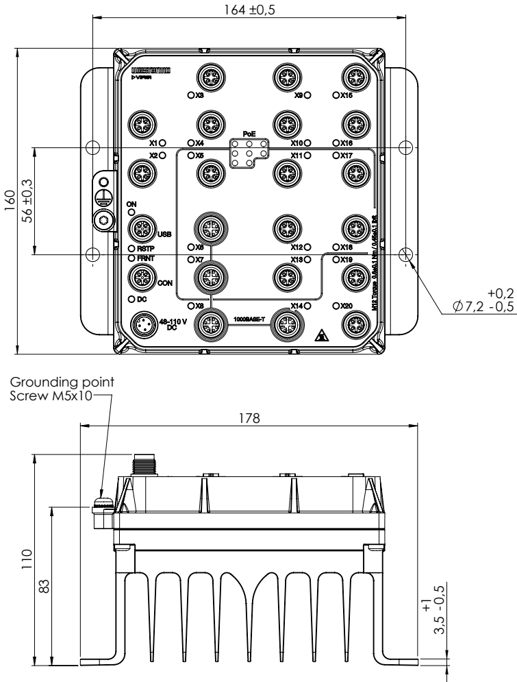
Abbildung 4. Maßzeichnung
