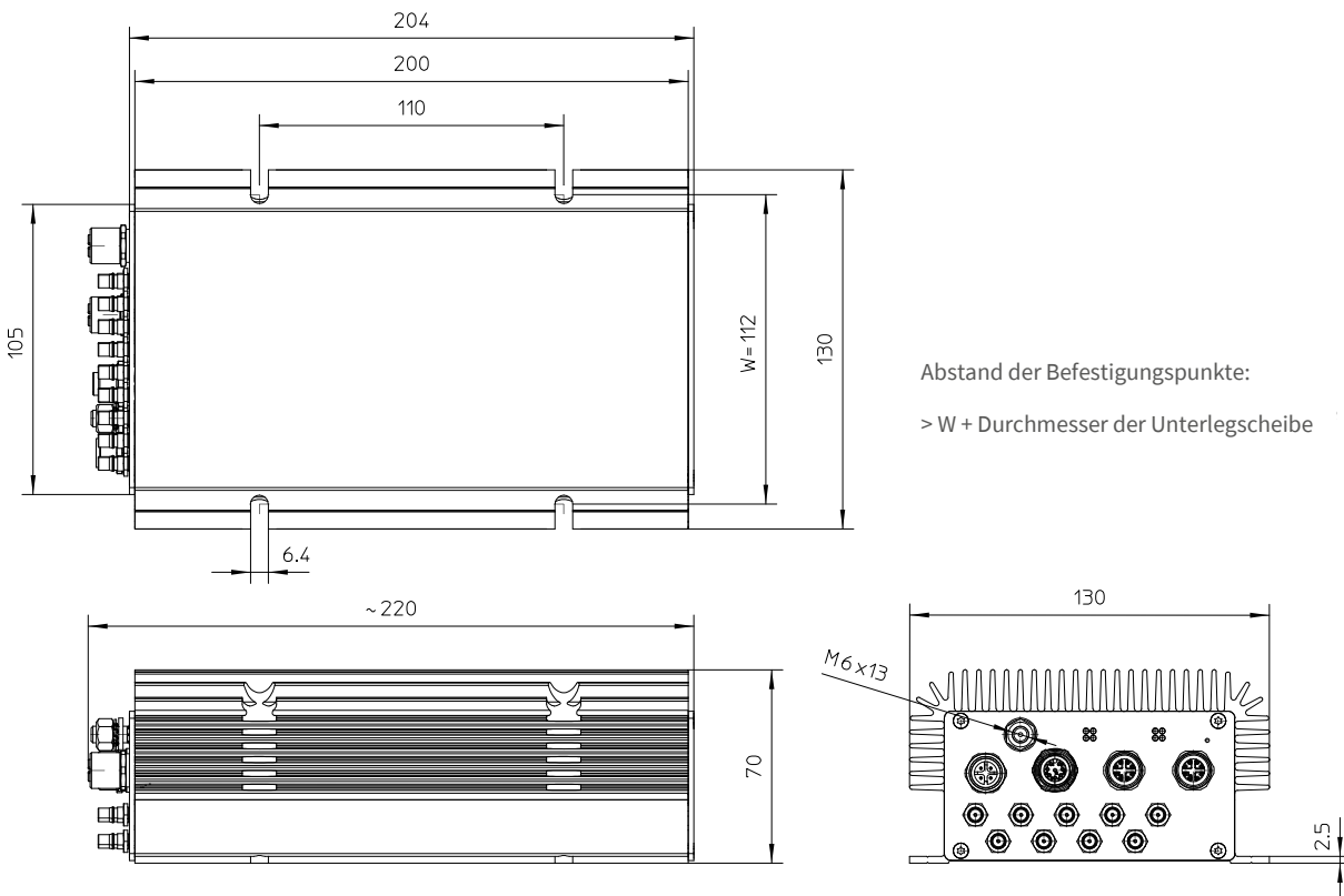
Figure 5 Abmessungen des CyBox AP 3- und CyBox RT 3-Gehäuses
