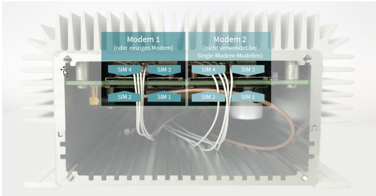
Figure 4 Belegung der SIM-Steckplätze pro Modem der CyBox RT 3
