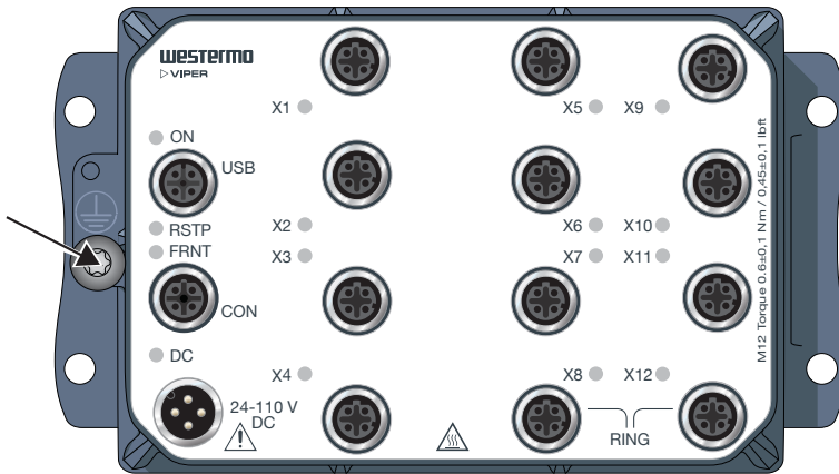
Abbildung 6. Erdungsanschluss
