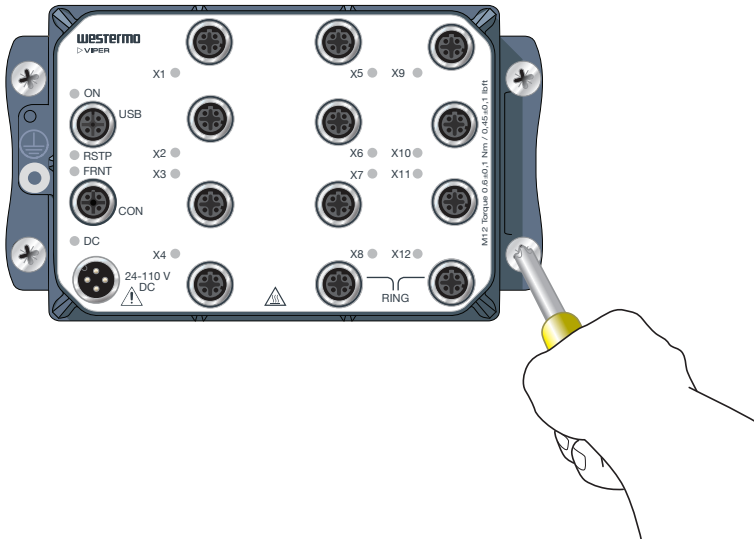
Abbildung 5. Wandmontage
