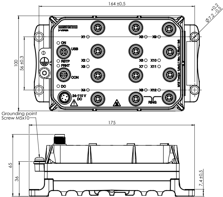
Abbildung 4. Maßzeichnung
